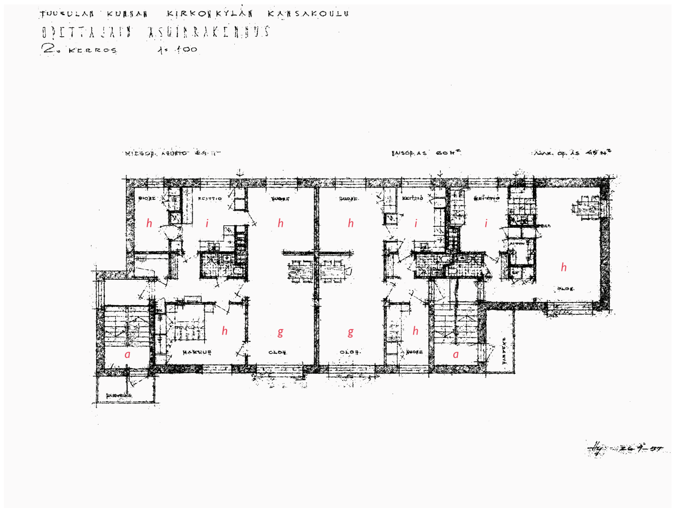
Yllä: kuva 60. Ote, opettajain asuinrakennus, 2. kerros 1:100, (Rakennustöimistö Heikki Siikonen 26.9.1957), pienennös
