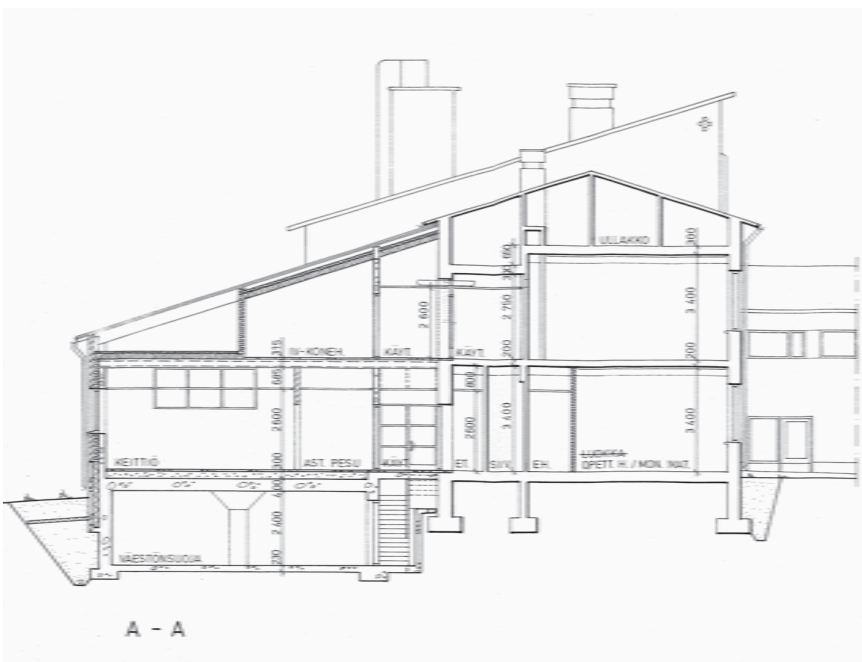
Yllä ja oikealla: kuva 41, 42 ja 43. Ote, leikkaus A-A, B-B ja G-G, ARK 1564 04.01, 1:100 (1.6.1989 Arkkitehtitoimisto Kaupunkisuunnittelu Oy), pienennös
