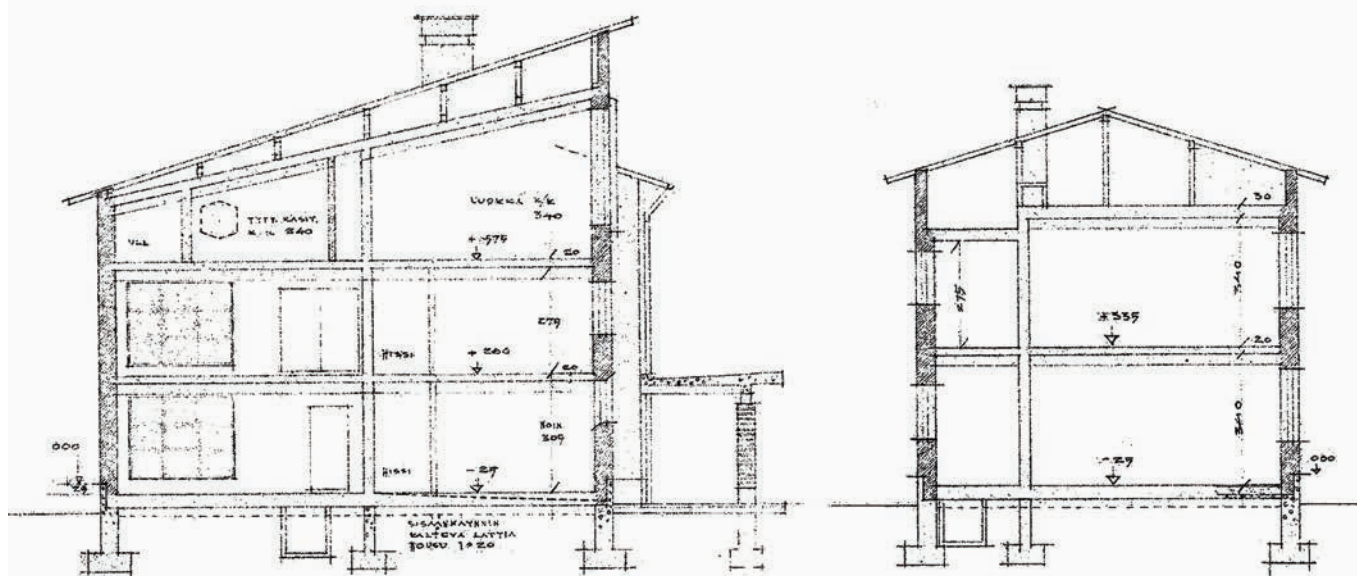
LEIKKAUS LUOKKIEIN KOHDALTA
