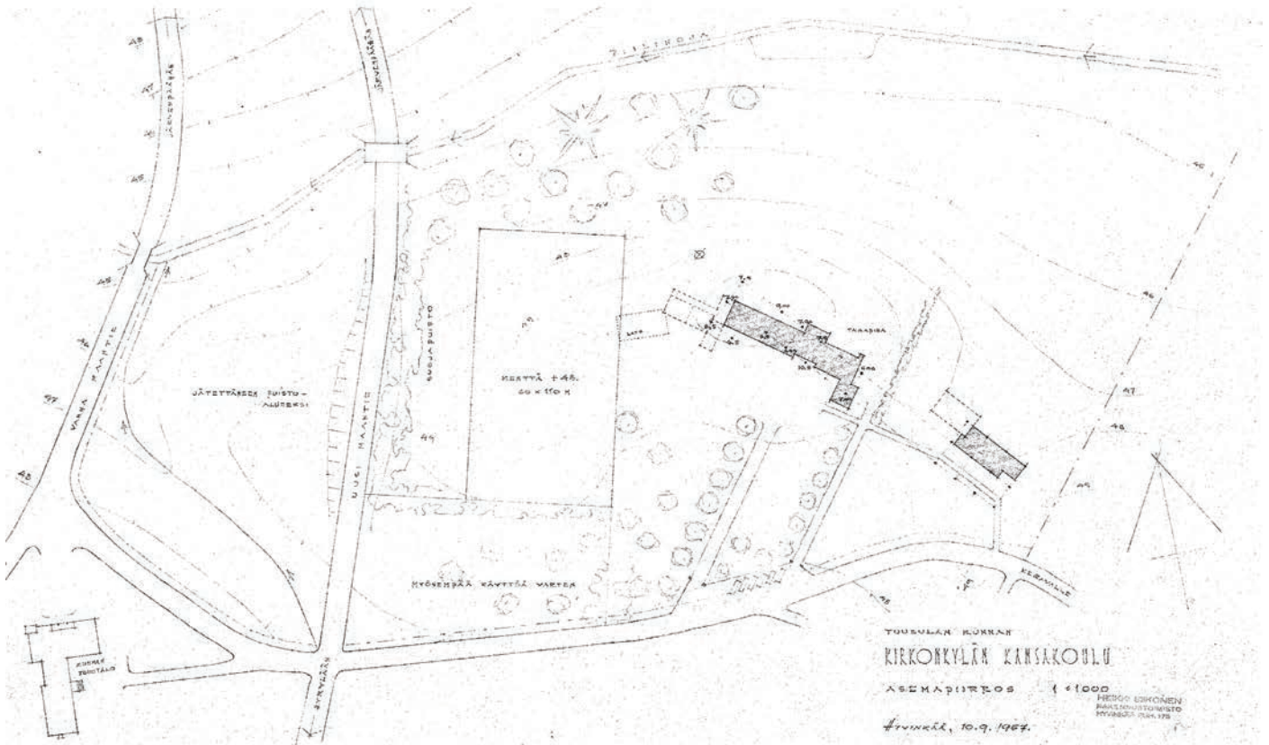
Yllä: kuva 53. Asemapiirustus 1:1000, (Rakennustoimisto Heikki Siikonen 10.9.1957), pienennös. Asemapiirustukseen on hahmoteltu laajennusosat koulurakennukselle ja asuintalolle, lato sekä pääsisäänkäynnille johtava puiden reunustama kuja, jotka ovat jääneet toteuttamatta
