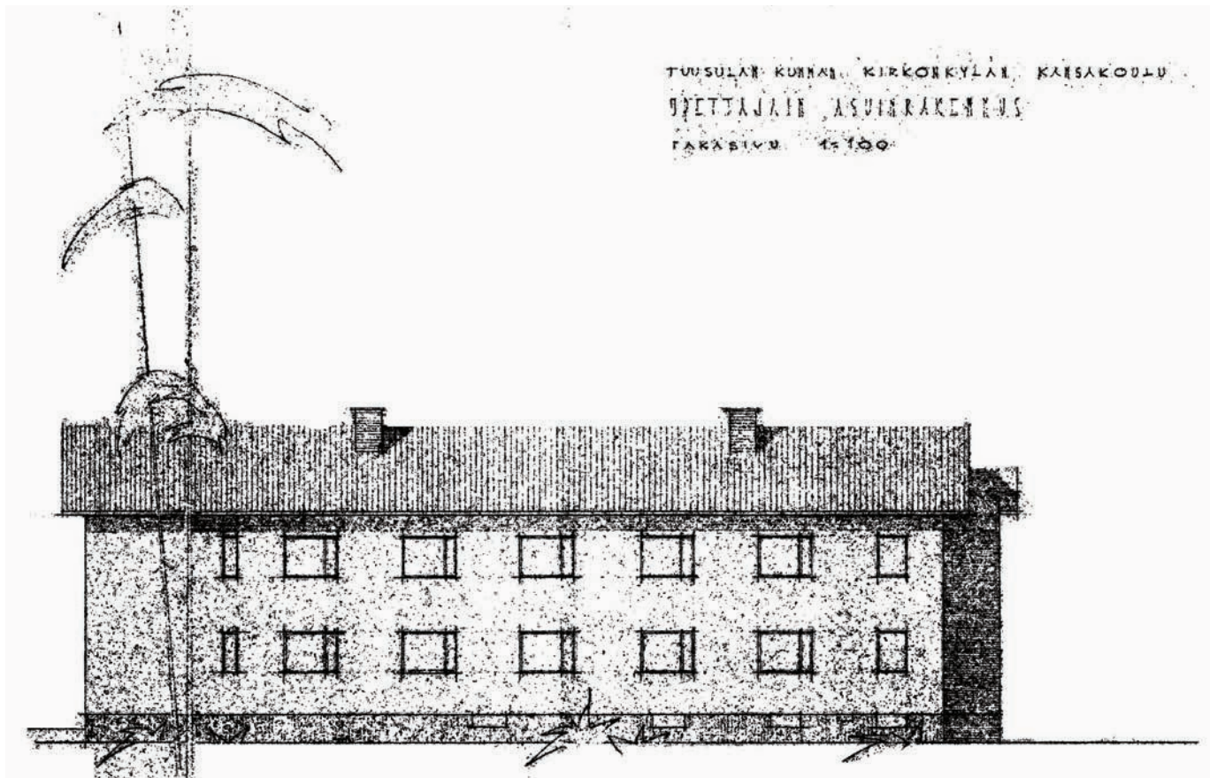
Yllä: kuva 57. Ote, opettajain asuinrakennus, julkisivu takaa 1:100, (Rakennustoimisto Heikki Siikonen 26.9.1957), pienennös
