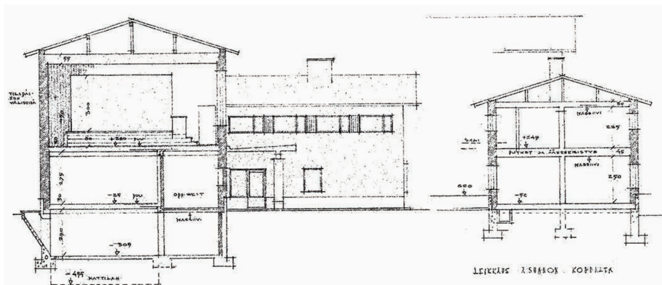
LEIKKAUS VOIMISTELUSALIN KOHDALTA
