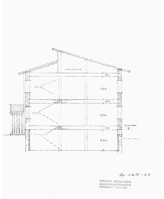
Yllä: kuva 56. Ote, opettajain asuinrakennus, päädyt ja leikkaus 1:100, (Rakennustoimisto Heikki Siikonen 26.9.1957), pienennös
